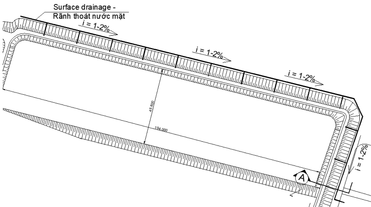
Hình 7. Mặt bằng bố trí rãnh thoát nước
