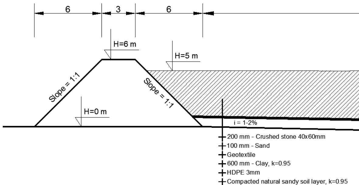
Hình 2. Cấu trúc hiện tại tại bãi chôn lấp rác Quảng Lợi
