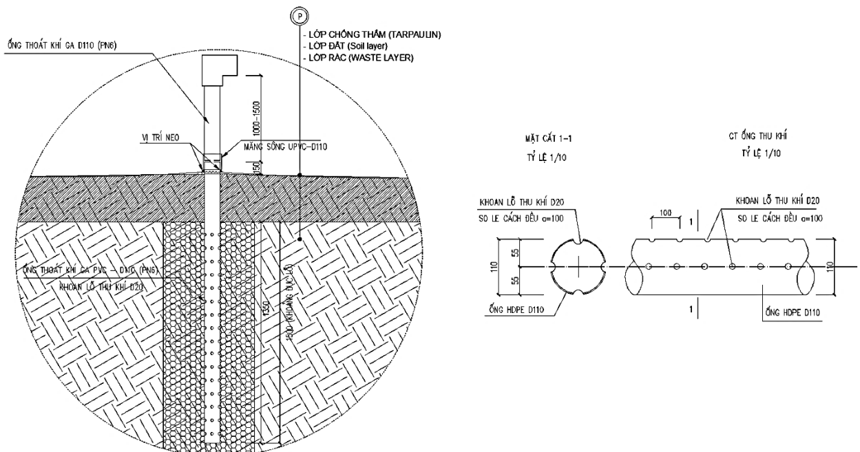
Hình 5. Chi tiết giếng thu khí
