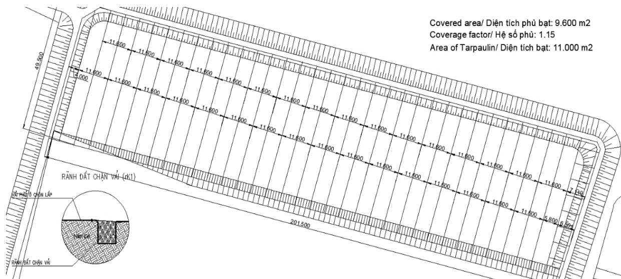
Hình 6. Mặt bằng trải bạt
